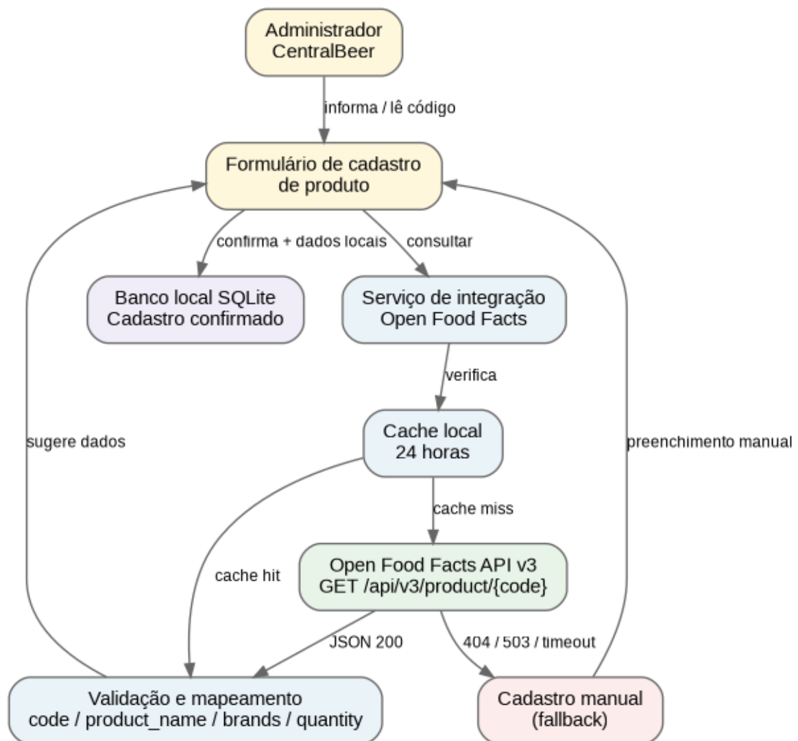
Figura 1 - Fluxo planejado da integração entre o CentralBeer e o Open Food Facts.
